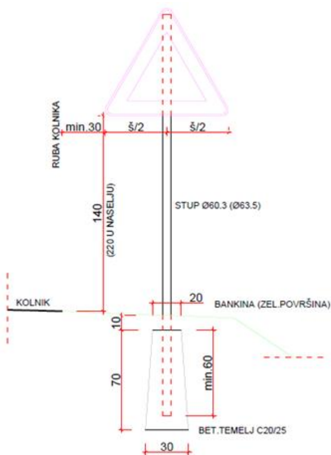
Detalj postavljanja prometnog znaka A39.
