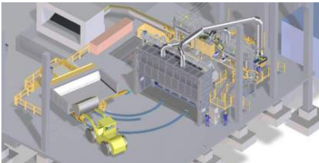
Slika 1./9. Jednokaturna talionička peć
