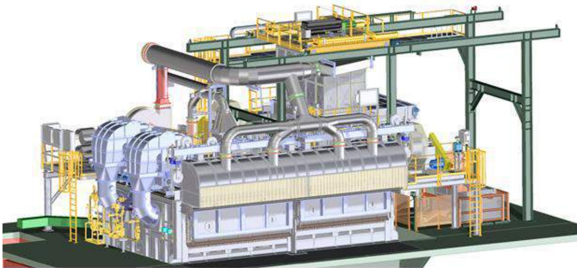
Slika 1./8. Višekomorna talionička peć
