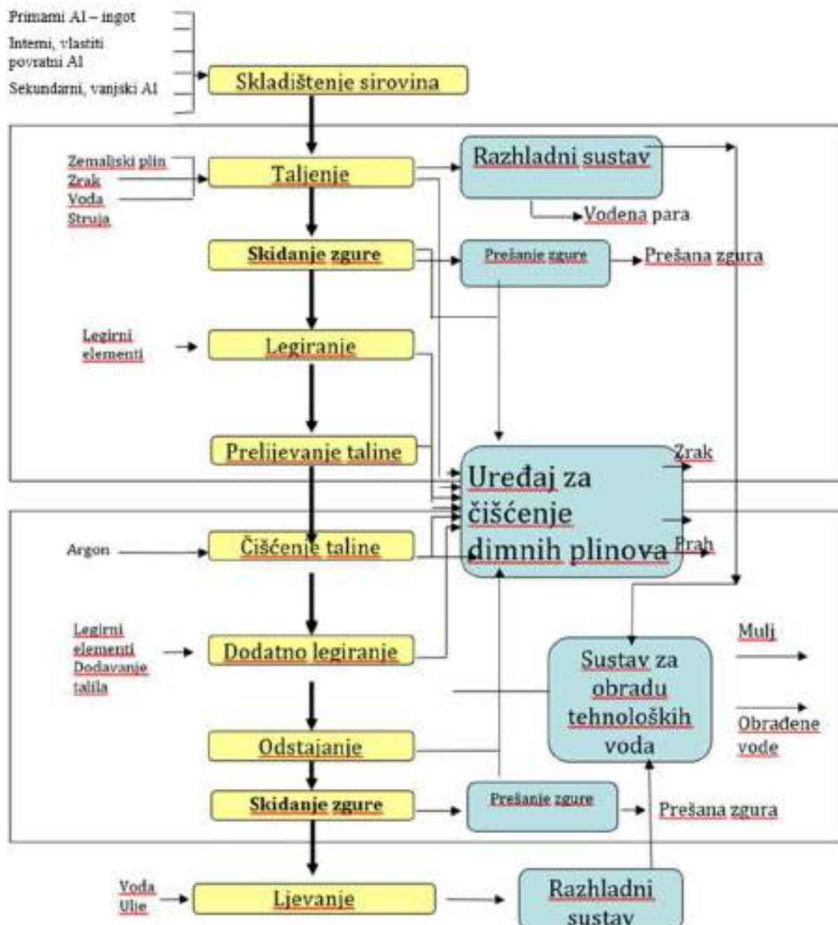
Slika 1./7. Shematski prikaz procesa
