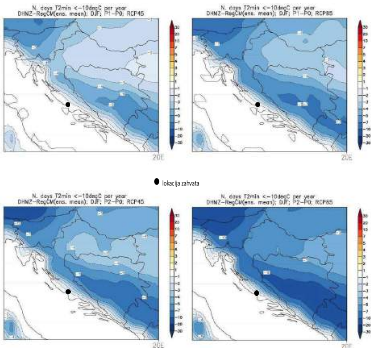
Slika 3./28. Promjene srednjeg broja ledenih dana (dan kada je minimalna temperatura manja ili jednaka -10°C) u odnosu na referentno razdoblje 1971.-2000. u srednjaku ansambla iz četiri integracije RegCM modelom. Lijevo: scenarij RCP4.5; desno: scenarij RCP8.5. Prvi red: promjene u razdoblju 2011.-2040. godine; drugi red: promjene u razdoblju 2041.-2070. godine. Mjerna jedinica: broj događaja u godini. Sezona: zima. [3]
