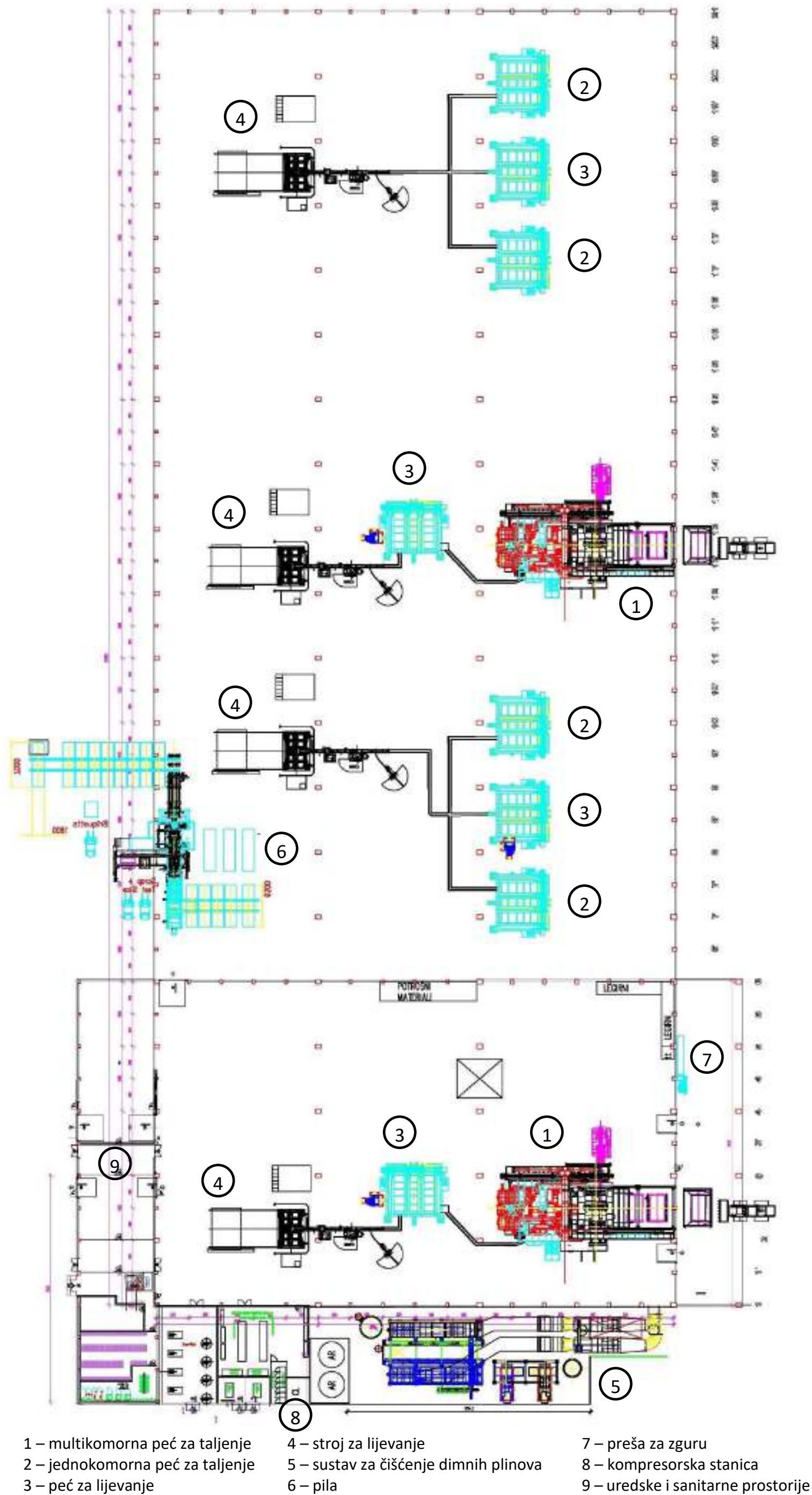
Slika 1./11. Shematski prikaz nove ljevaonice [1]
